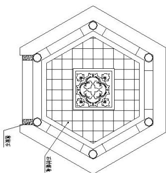
平面
